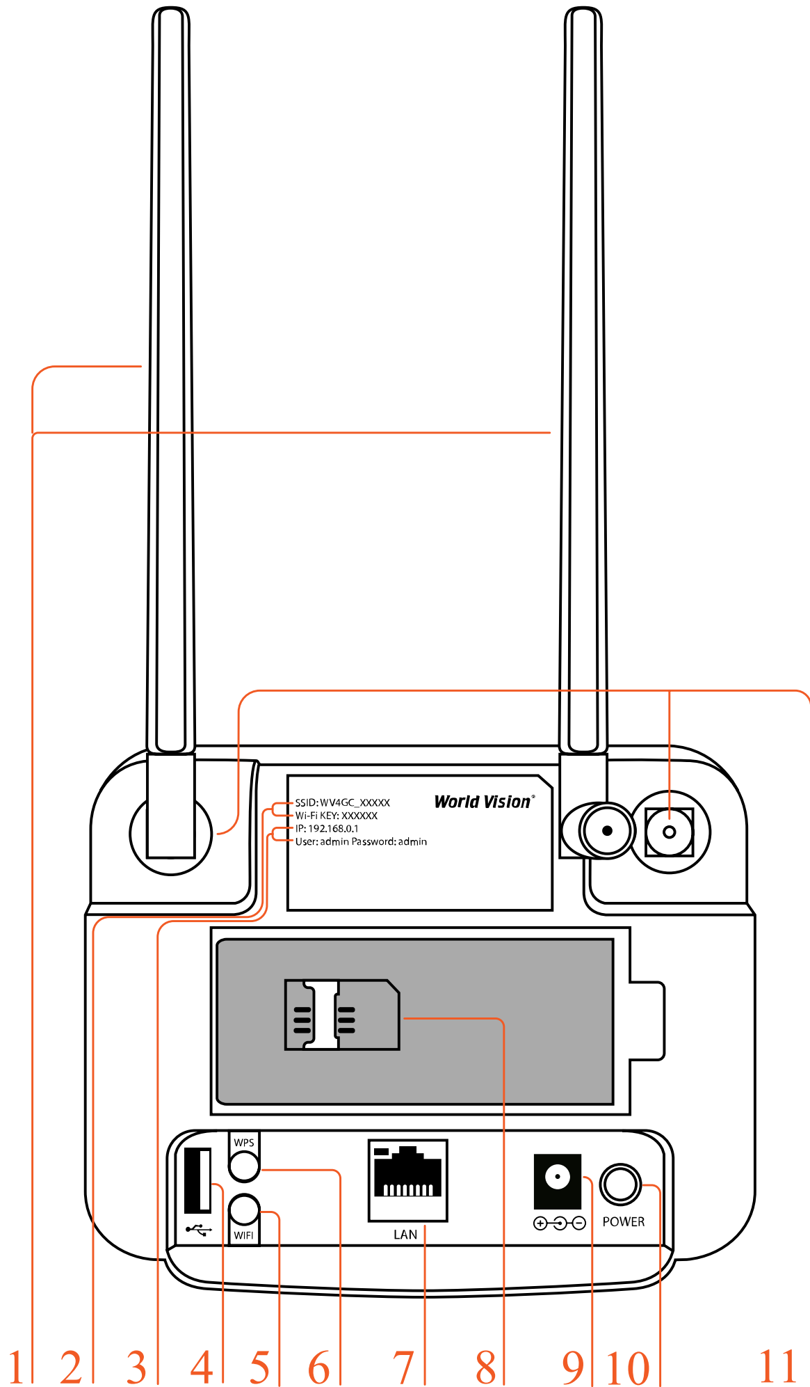
1. Знімні 4G LTE антени тип конектора SMA (male)
